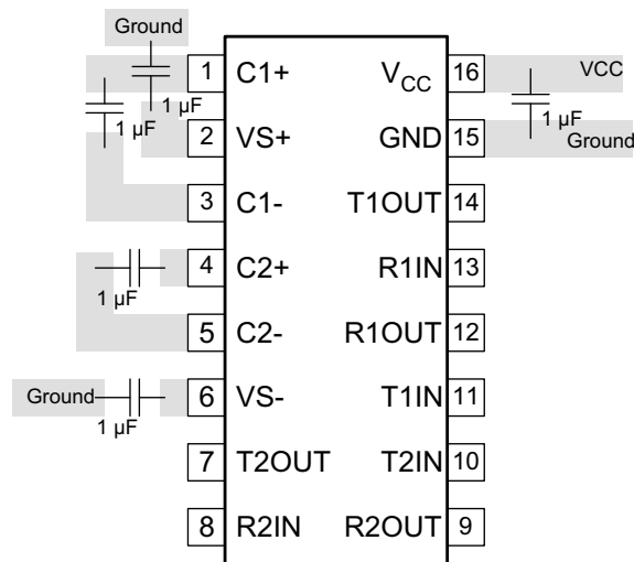
図 8-4. Layout Schematic
