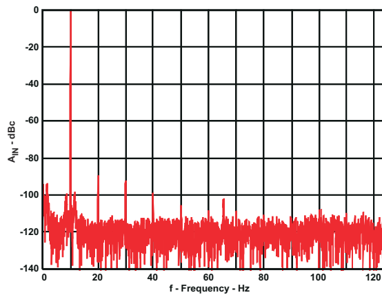
图 9-10. ADS8326 and OPA836 10-kHz FFT
