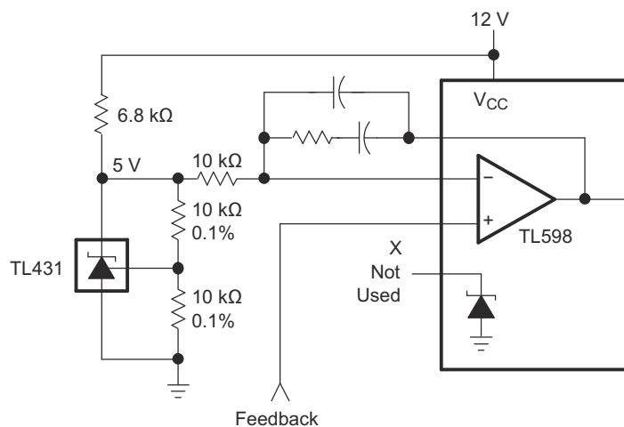
図 9-11. 基準電圧内蔵 PWM コンバータ
