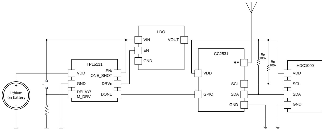
簡略化されたアプリケーション回路図
