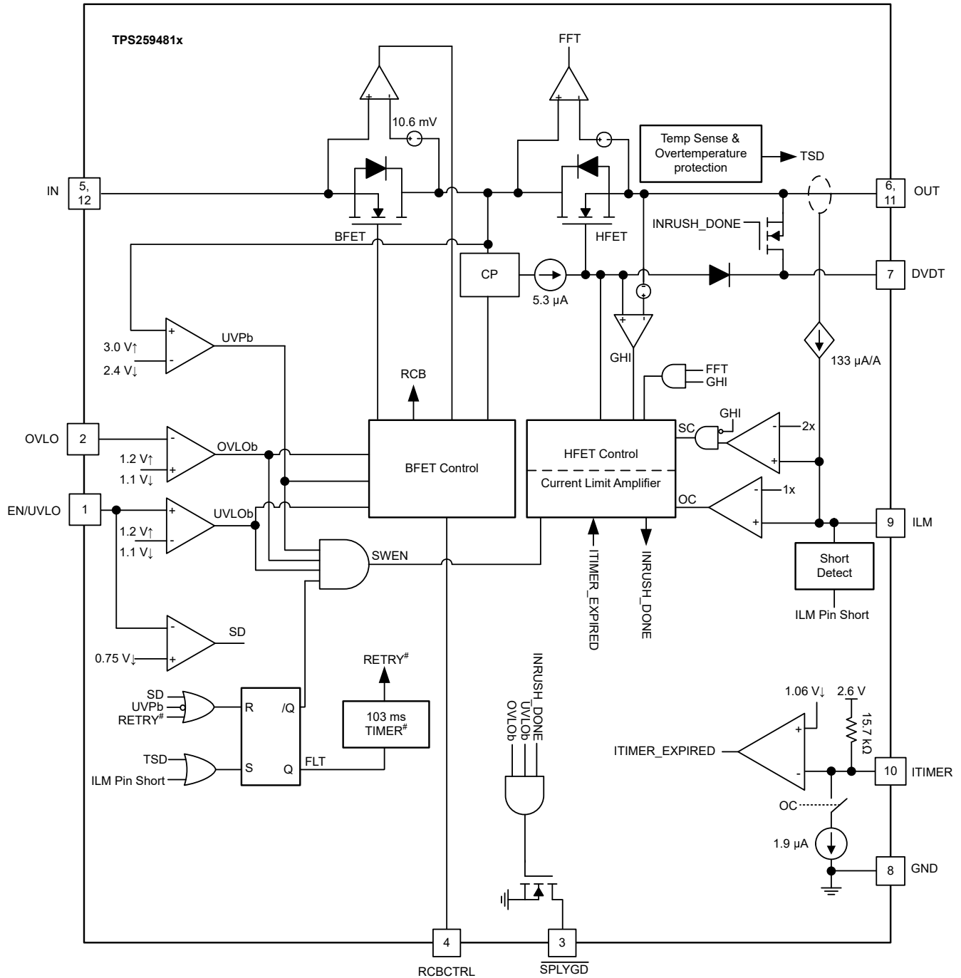
図 8-2. TPS25948x Block Diagram
