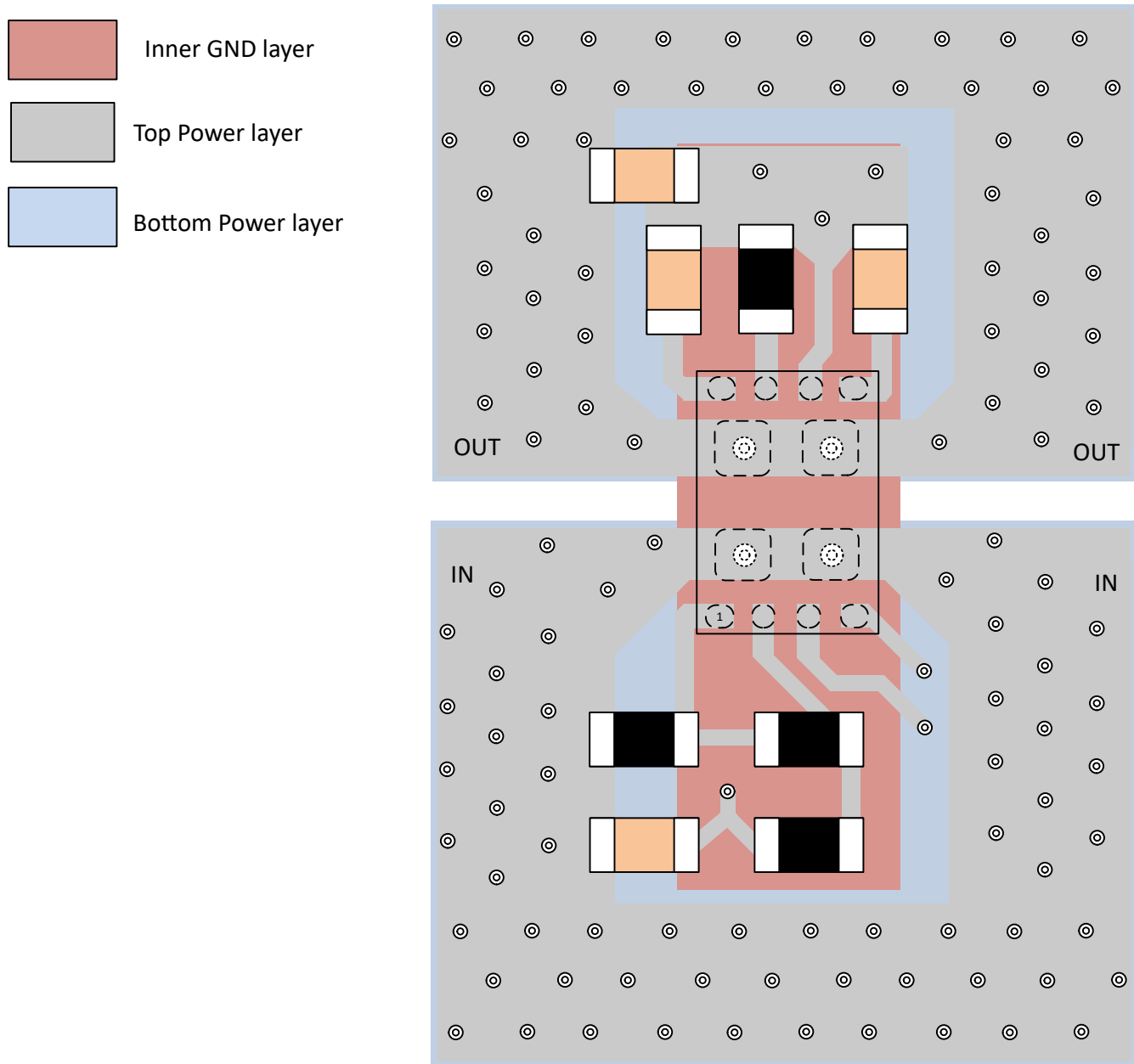
図 9-24. Layout Example
