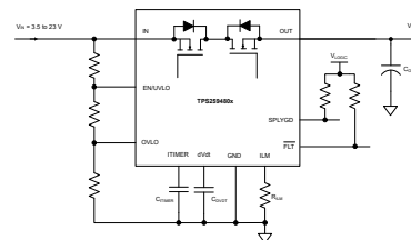
概略回路図
