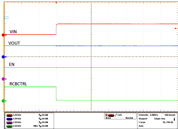
図 9-10. Power Up in OTG Mode
