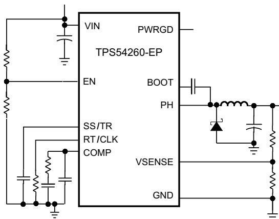
概略回路図
