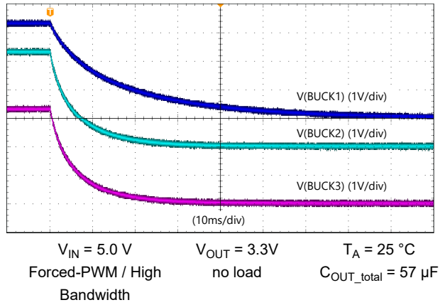
8-8. Bucks Discharge
