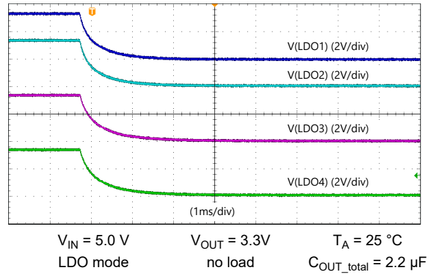
8-9. LDOs Discharge
