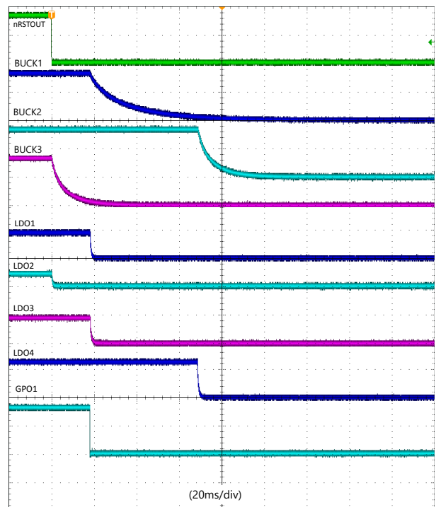
8-9. LDOs Discharge
