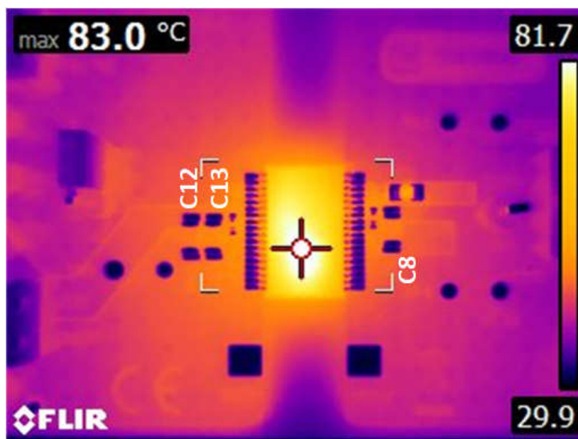
图 12-25. Thermal Image
