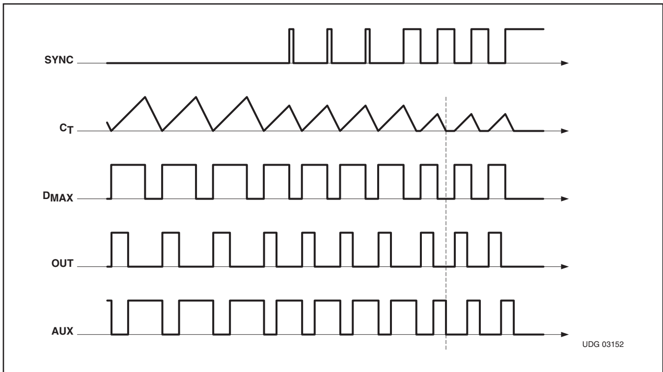
図 6. Synchronization Waveforms
