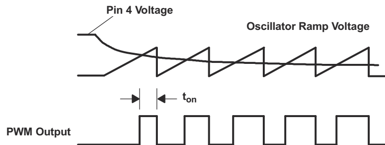
図 10-5. ソフトスタート回路
