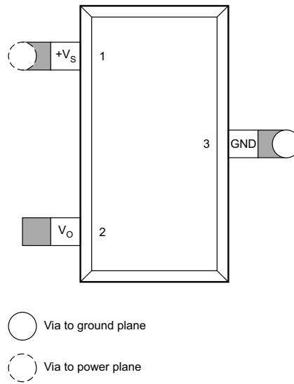
図 8-8. PCB Layout
