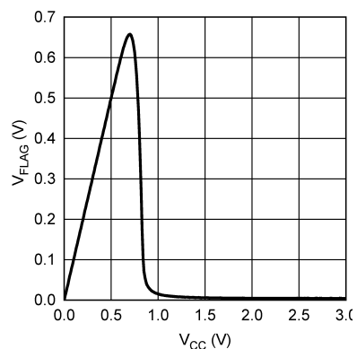
図 6-9. フラグ電圧と電源電圧との関係
