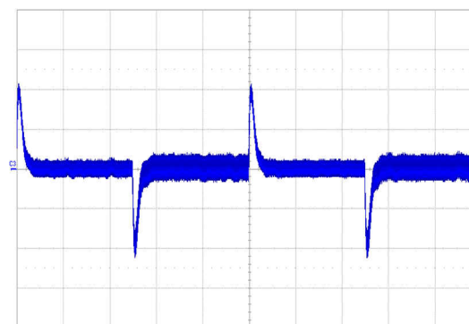
图 9-5. Load Transient
