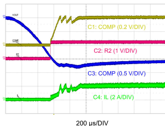
图 9-4. Automatic Wake-Up
