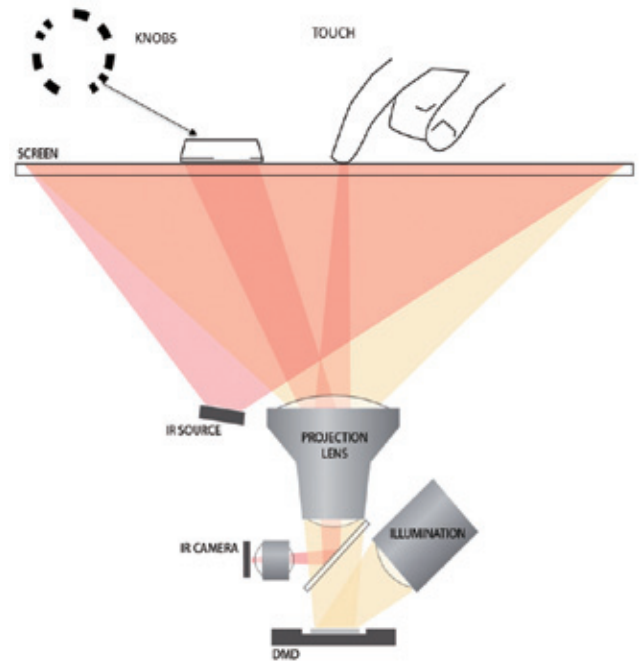
システム・ブロック図: DLP 双方向型ディスプレイ
