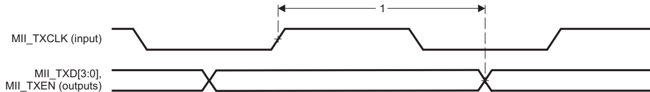
Figure 5-129. PRU-ICSS MII_TXD[3:0], MII_TXEN Timing
